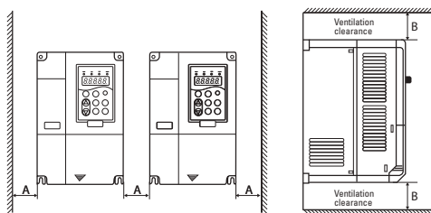
Рис. 4-1 Монтажная схема
