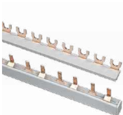
Шины соединительные типа FORK («вилка») и PIN («гребенка») EKF PROxima
