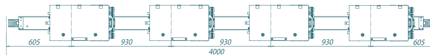
Отводный блок ОБ-630
