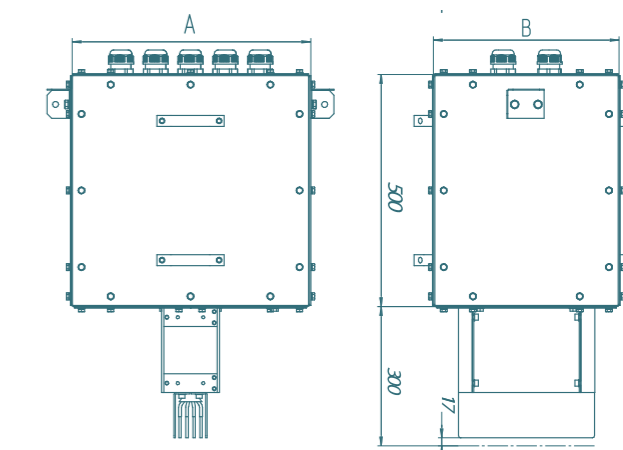
Чертеж кабельный ввод IP 55
